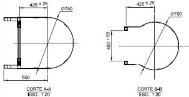
Detalhes do guarda-corpo
